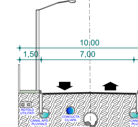
SECTIUNE B - B'
