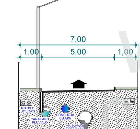
SECTIUNE A - A' * SD APLICA PDNTRU TOATE STRAZILE CU SENS UNIC EXCPTAND STR. BABA NOVAC SI STR. B.S. DELAVRANCEA
